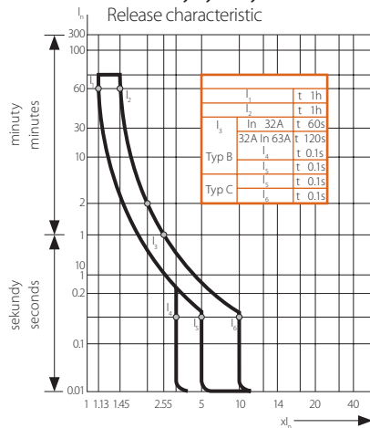
Charakterystyka wyzwalania Release characteristic
